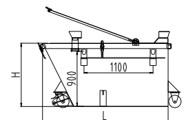
UG 30 S/U stapelbar, mit Rollen
